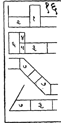
१६. Quoin brick, Squint brick : कोपऱ्यांची वीट मांडणी.
